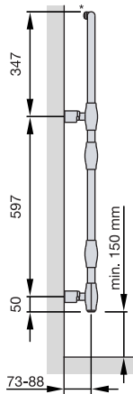
Zijaanzicht:
