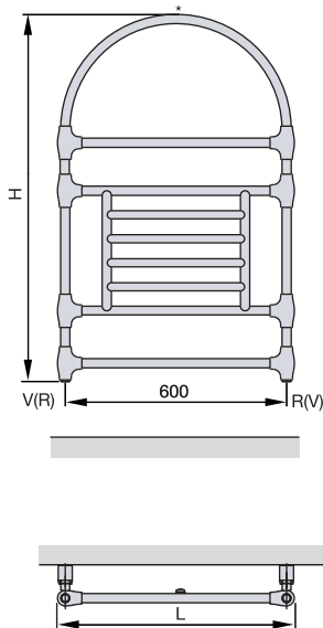
Vooraanzicht:
